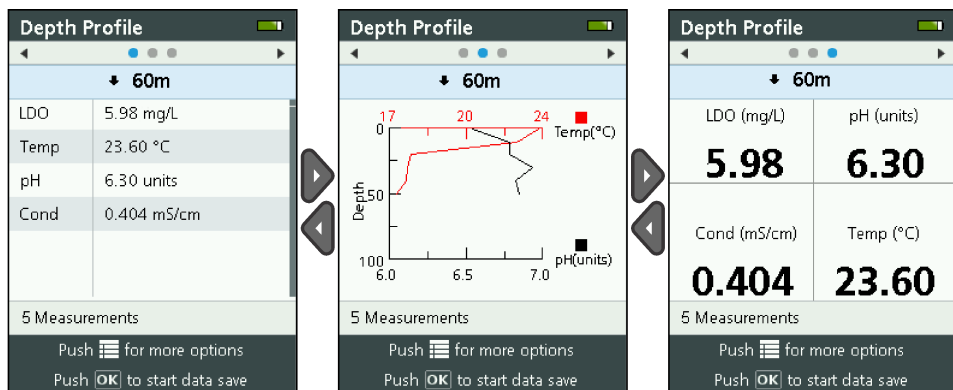
图 9 深度剖面监测视图
