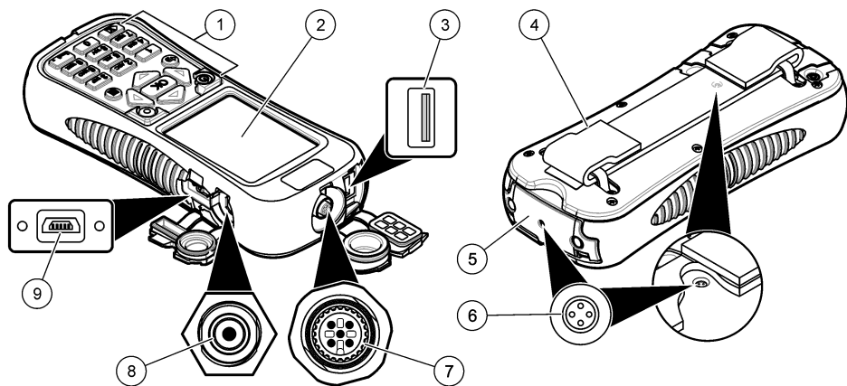
图 1 仪器概述
