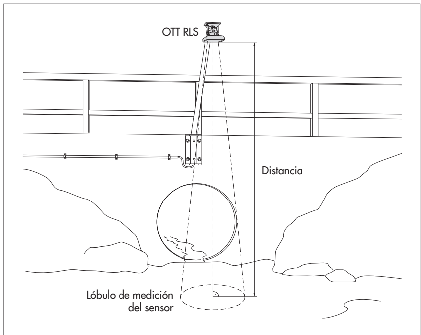
Fig. 3: Ejemplo de uso 2: Montaje de OTT RLS en una construcción auxiliar, por ejemplo, en un estribo metálico con placa de montaje.
