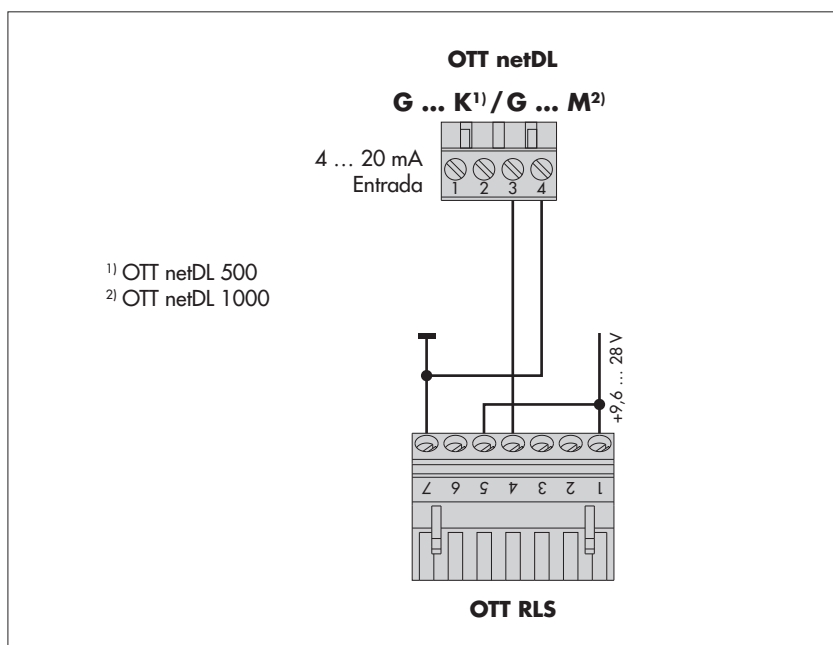
Fig. 12: Conexión del OTT RLS a OTT netDL mediante la interfaz 4 ... 20 mA.
