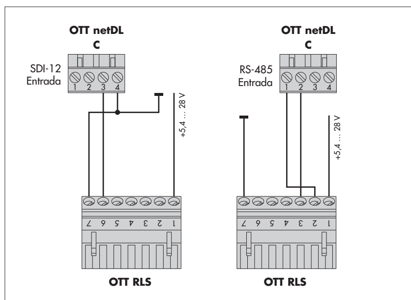
Fig. 10: Conexión de OTT RLS a OTT netDL mediante la interfaz SDI-12. Las letras sobre los elementos atornillados de emborne identifican las conexiones posibles a OTT netDL.
