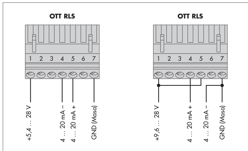
Fig. 7: Ejemplos para la conexión del OTT RLS mediante la interfaz de 4 ... 20 mA a un recolector de datos cualquiera.
