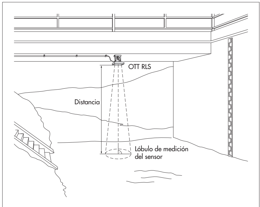
Fig. 2: Ejemplo de uso 1: Montaje de OTT RLS en un puente. La proyección del lóbulo de medición sobre la superficie del agua es aproximadamente circular.
