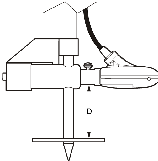
Abbildung 12 Offset-Abstand (D)
